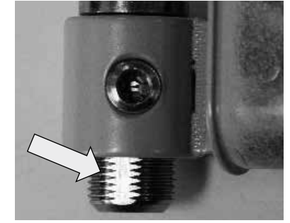
Beim Fixieren muss stets auf der abgefrästen Fläche des Höhentellers geklemmt werden!
