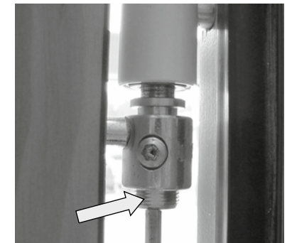
Fixierschraube lösen.
